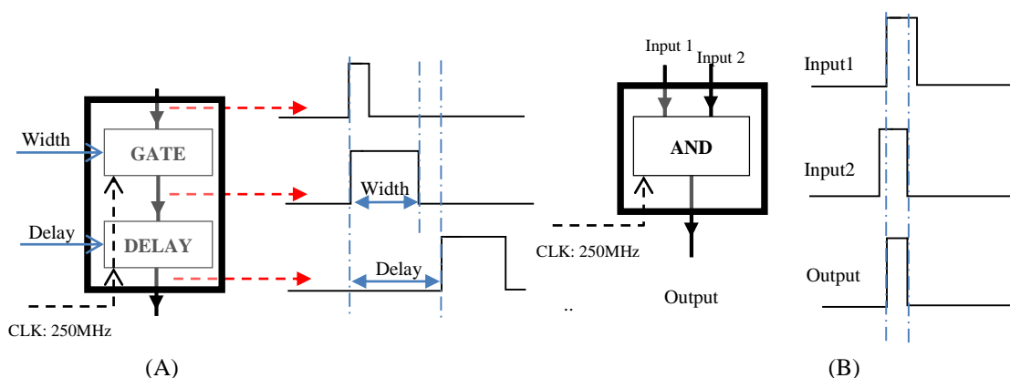
Hình 2. Sơ đồ khối của module Gate/delay (A) và module Coin (B) được phát triển bởi nhúng FPGA
