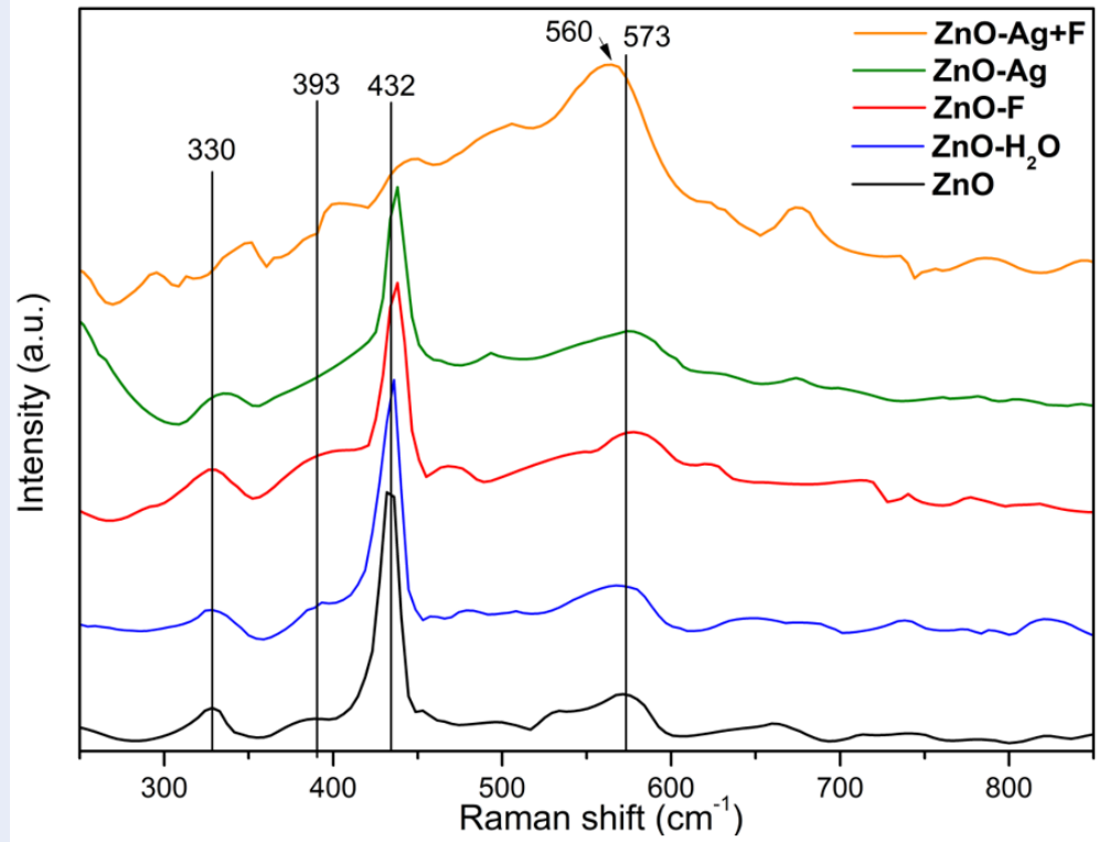
Hình 3: Phổ Raman của các mẫu màng mỏng ZnO không biến tính và mẫu màng mỏng ZnO được biến tính bề mặt.
