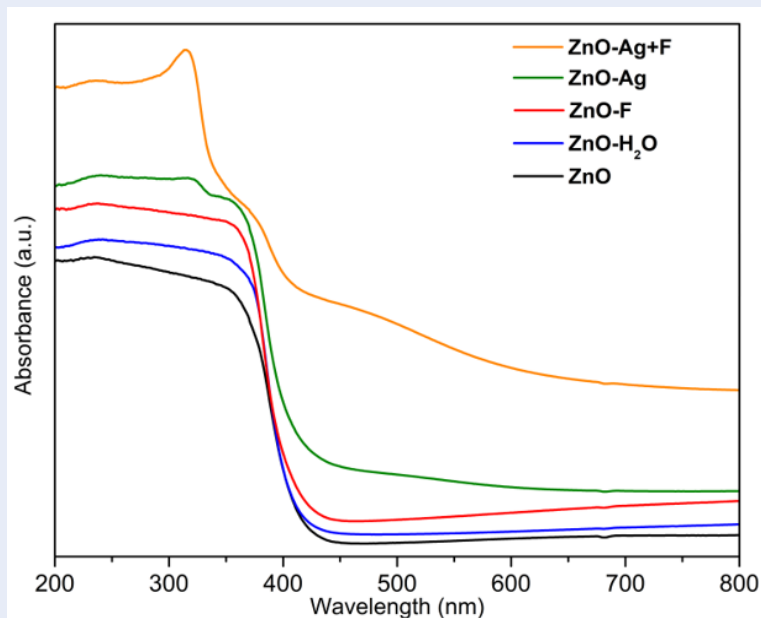
Hình 7: Phổ hấp thụ UV–khả kiến của các mẫu màng mỏng ZnO không biến tính và mẫu màng mỏng ZnO được biến tính bề mặt.
