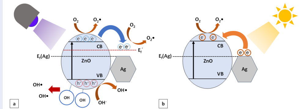
Hình 11: Sơ đồ cơ chế xúc tác quang hóa được đề xuất của các mẫu màng mỏng ZnO với sự hiện diện của các hạt Ag kim loại trong vùng UVA (a) và ánh sáng khả kiến (b).
