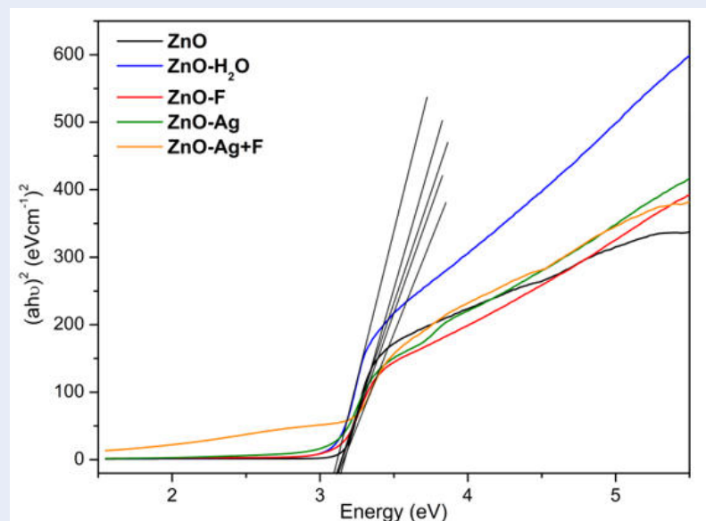
Hình 8: Biểu đồ Tauc của các mẫu màng mỏng ZnO không biến tính và mẫu ZnO biến tính bề mặt.
